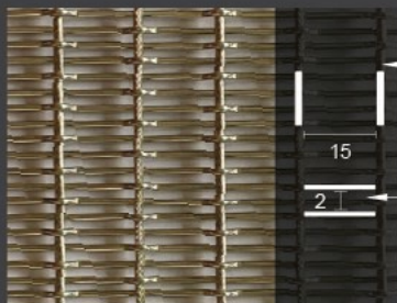
21. BM-M7521 (5.2 kg. / sqm.)
